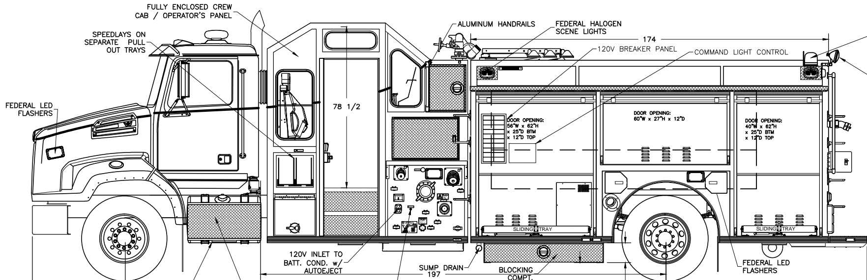
LEFT SIDE
