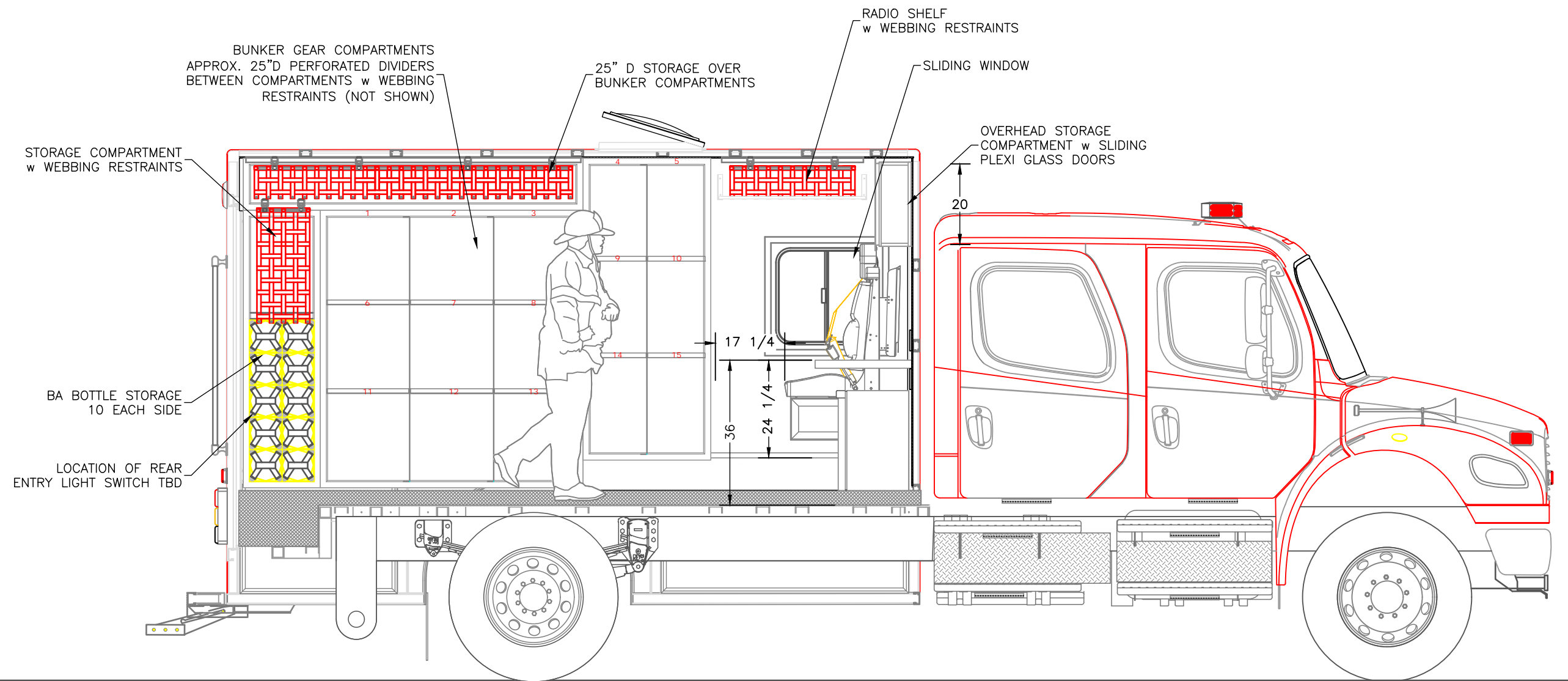
SECTION A-A
